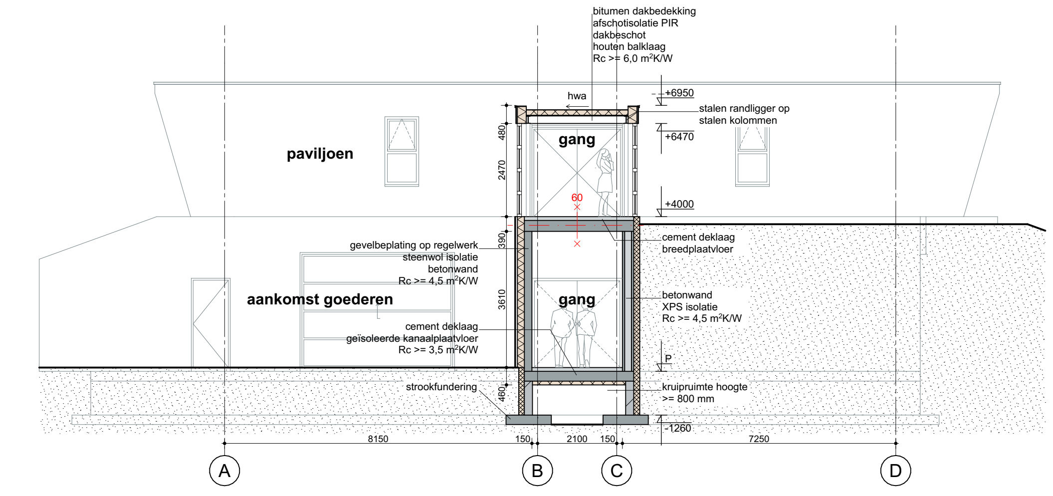
doorsnede D-D
