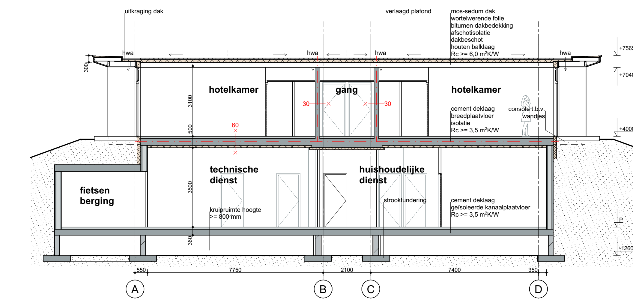
doorsnede E-E
